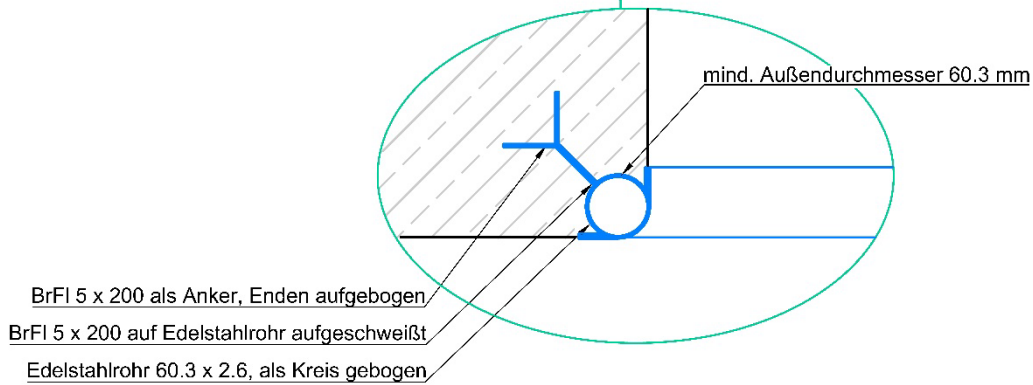
Schnitt B-B
