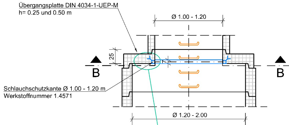
Schnitt A - A
