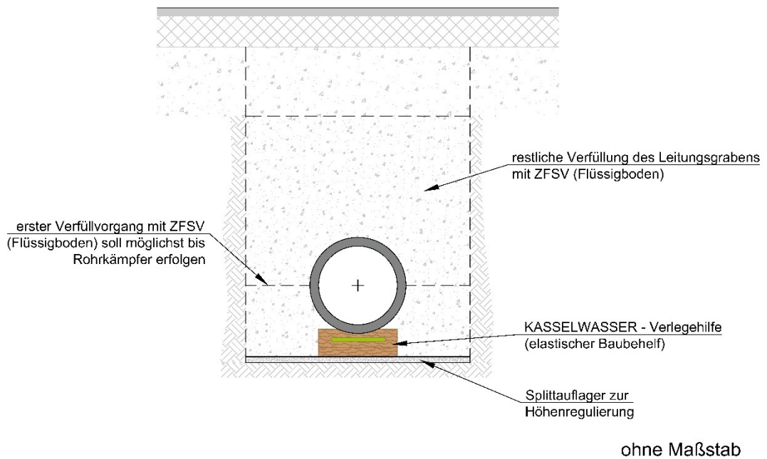
Abbildung 5: Querschnitt des Leitungsgrabens nach vollständigem Einbau des Abwasserkanals
