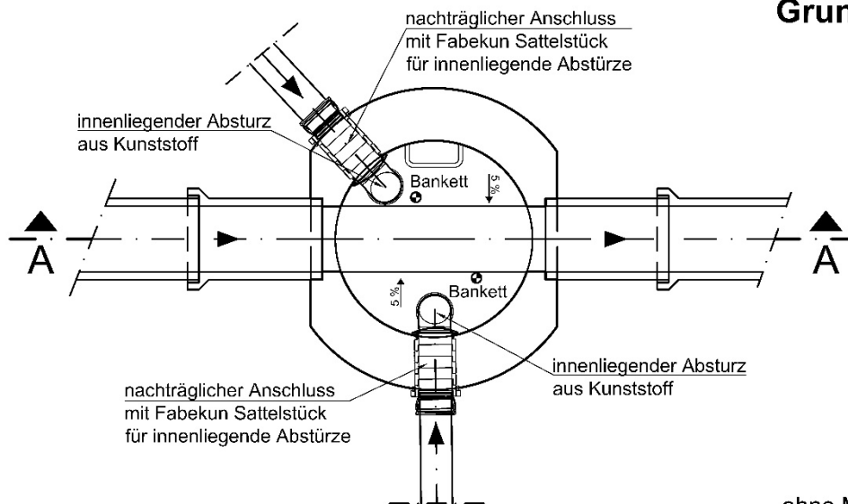
Grundriss
