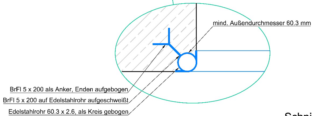
Schnitt B - B (UK Decke)
