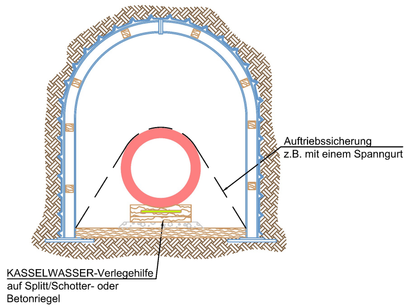
Abbildung 17: Querschnitt Lagefixierung des Rohres Typ 1
