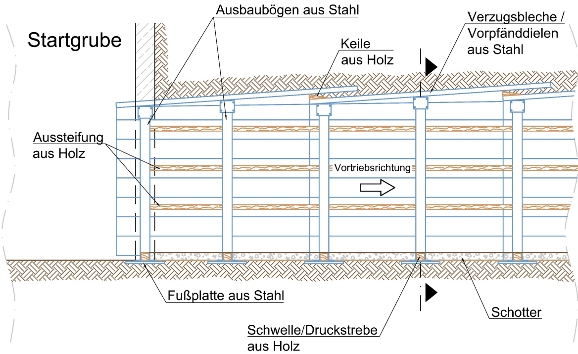
Abbildung 11: Längsschnitt Stollenbau mit Stahlverzug
