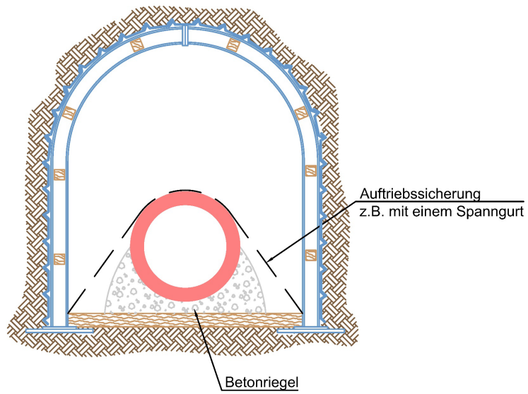
Abbildung 19: Querschnitt Lagefixierung des Rohres Typ 3
