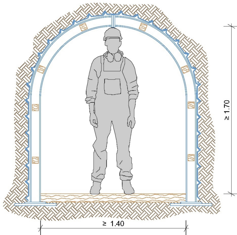
Abbildung 25: Querschnitt Mindestlichtmaße für den Arbeitsplatz im Stollen mit Stahlverzug (in Stollen mit Holzverzug analog)
