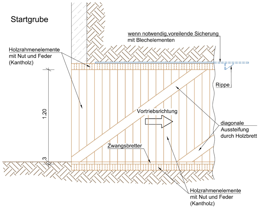
Abbildung 15: Längsschnitt Pionierstollen
