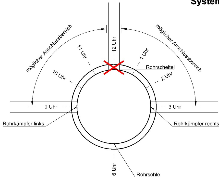
Abbildung 6: möglicher Anschlussbereich von Abwasserleitungen an Abwasserkanäle
