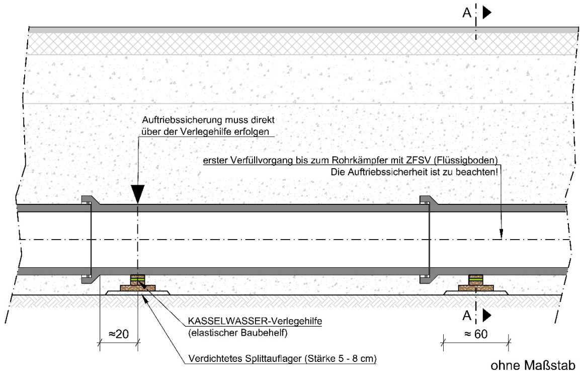
Abbildung 4: Längsschnitt des Leitungsgrabens nach vollständigem Einbau des Abwasserkanals
