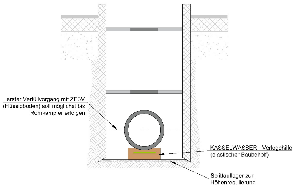
Abbildung 3: Lagefixierung des Abwasserrohres auf KASSELWASSER-Verlegehilfe
