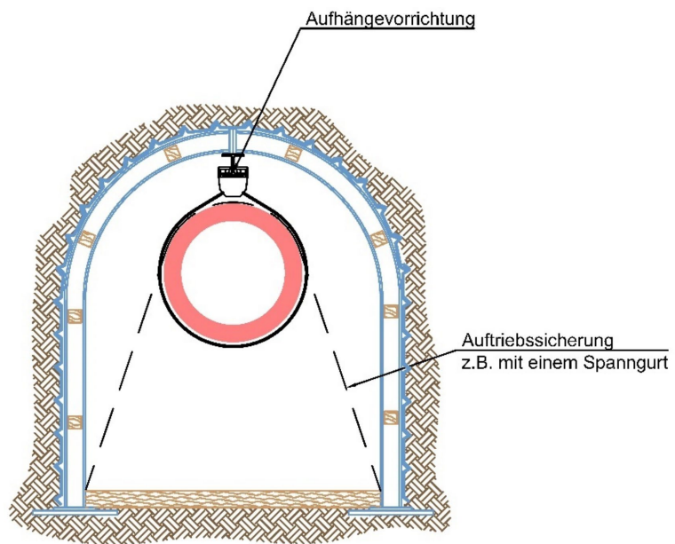
Abbildung 20: Querschnitt Lagefixierung des Rohres Typ 4
