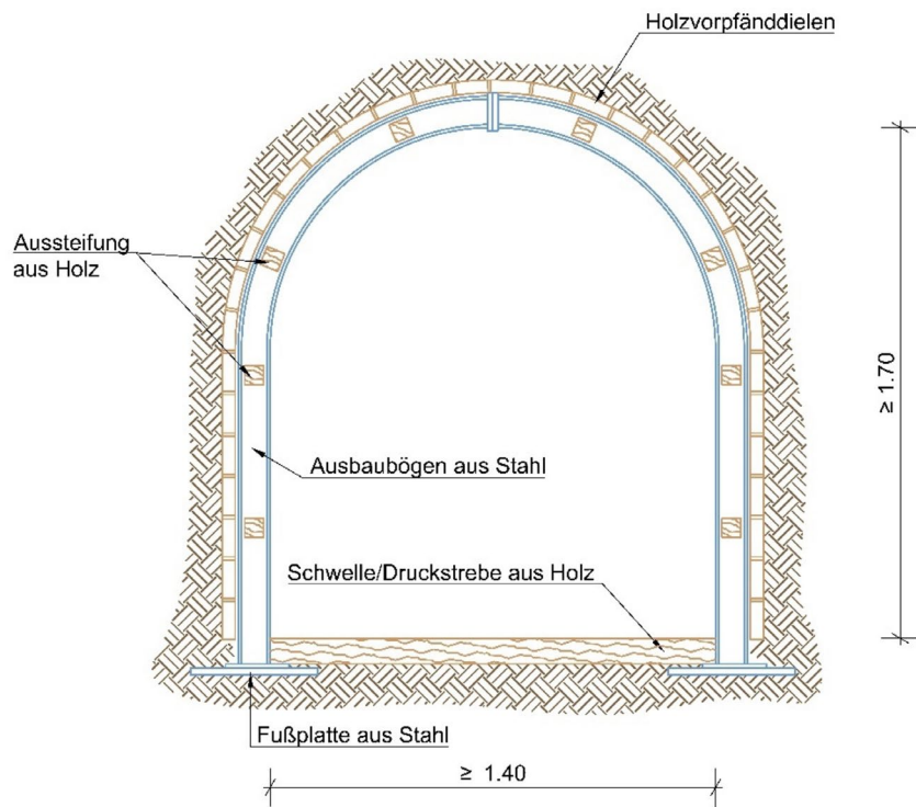
Abbildung 14: Querschnitt Stollenbau mit Holzverzug
