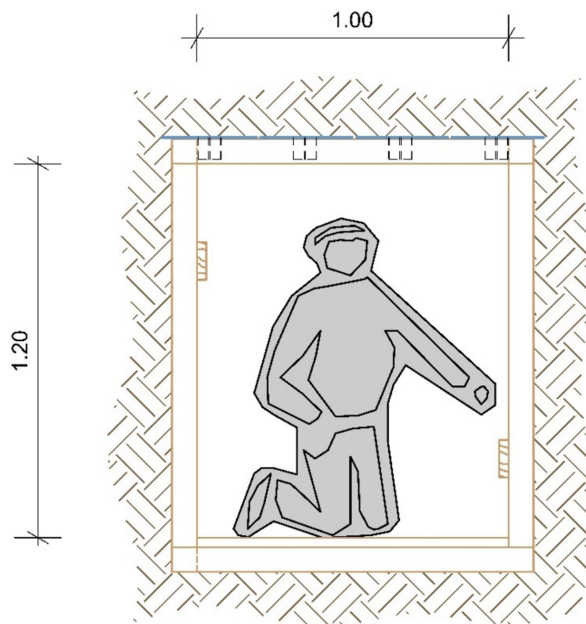
Abbildung 27: Querschnitt Mindestlichtmaße für Arbeitsplatz in Pionierstollen
