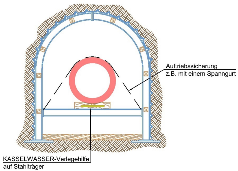
Abbildung 18: Querschnitt Lagefixierung des Rohres Typ 2
