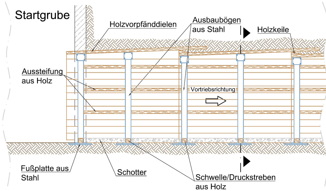
Abbildung 13: Längsschnitt Stollenbau mit Holzverzug
