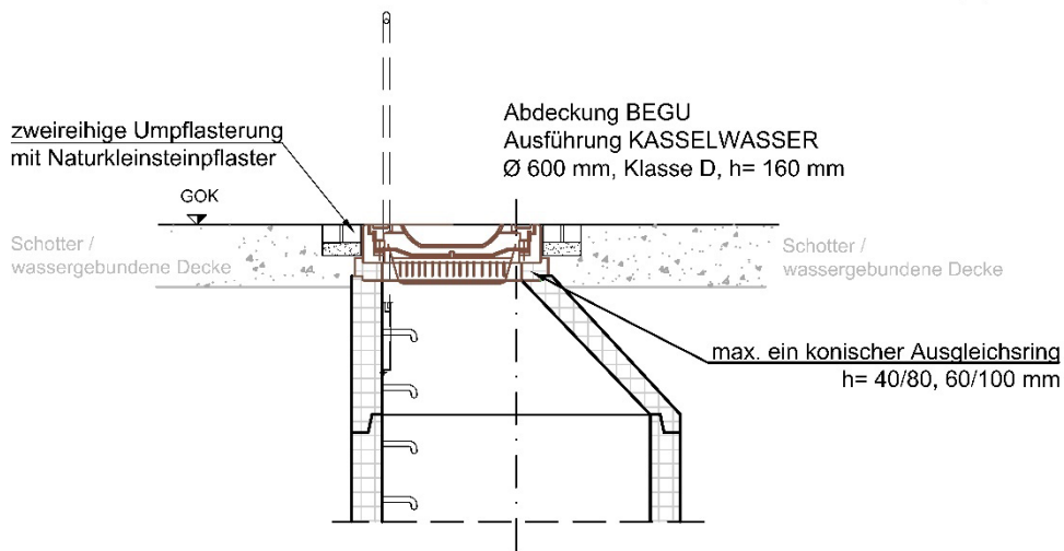
Schnitt B - B
