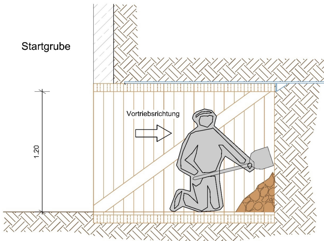
Abbildung 26: Längsschnitt Mindestlichtmaße für Arbeitsplatz in Pionierstollen
