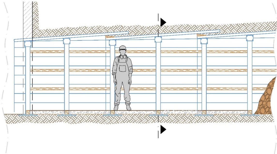
Abbildung 24: Längsschnitt Mindestlichtmaße für den Arbeitsplatz im Stollen mit Stahlverzug (in Stollen mit Holzverzug analog)
