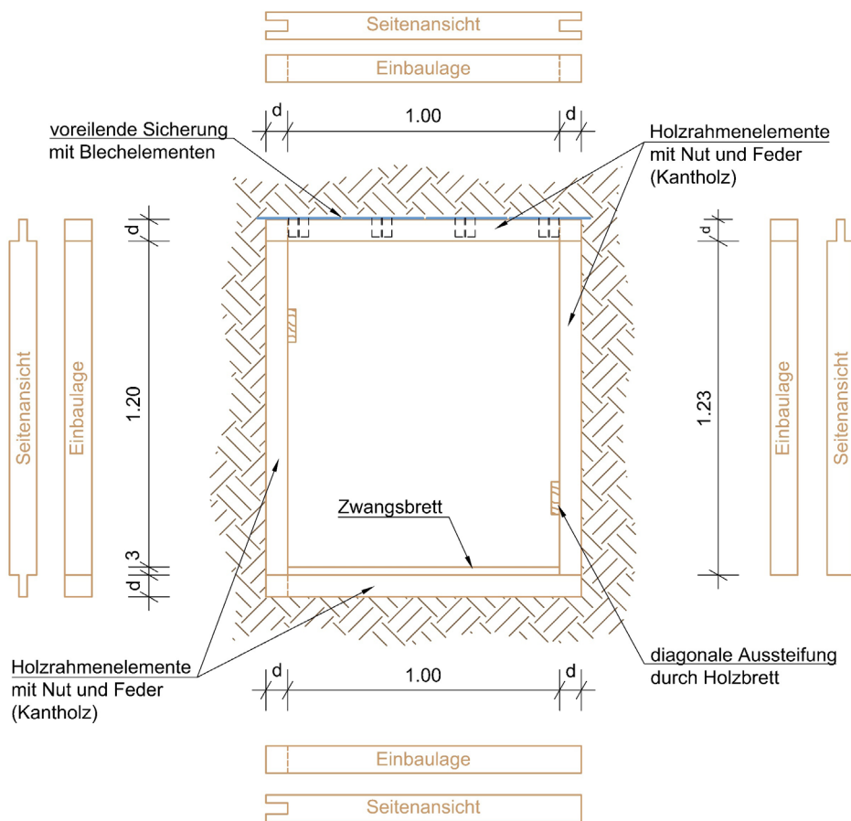
Abbildung 16: Querschnitt Pionierstollen
