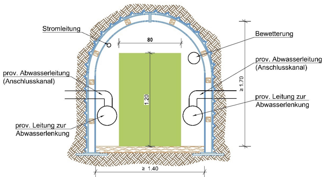
Abbildung 22: Querschnitt Mindestlichtmaß für Verkehrswege in Stollen mit Holz- und Stahlverzug
