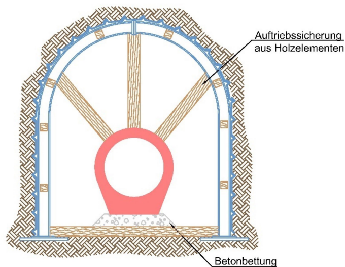
Abbildung 21: Querschnitt Lagefixierung des Rohres Typ 5
