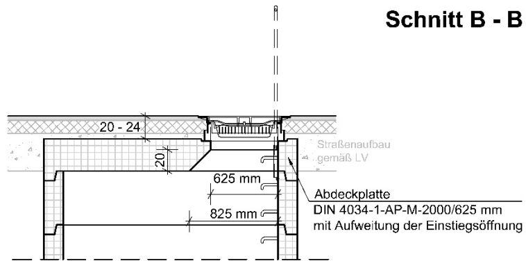
Schnittdarstellung Schematisch
