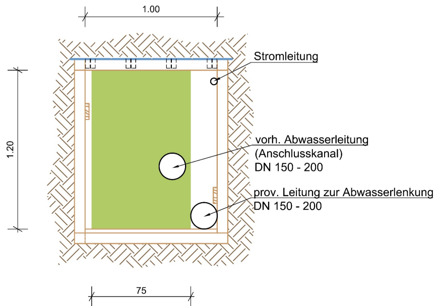
Abbildung 23: Querschnitt Mindestlichtmaße für Verkehrswege in Pionierstollen
