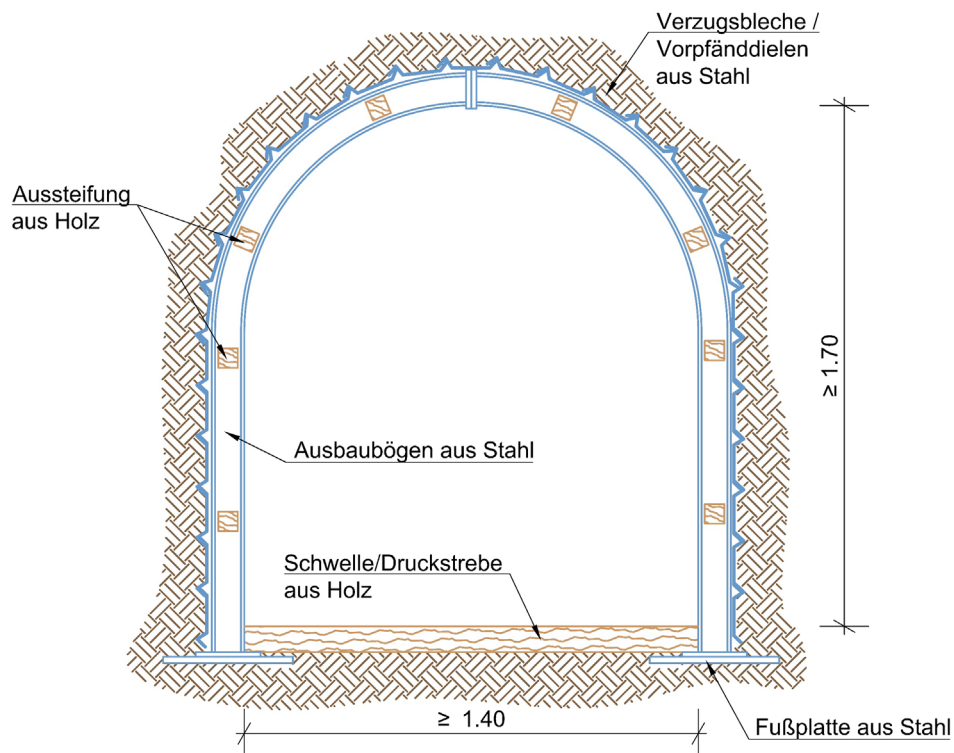
Abbildung 12: Querschnitt Stollenbau mit Stahlverzug
